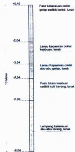
DETAIL BM.5 P.4+800
