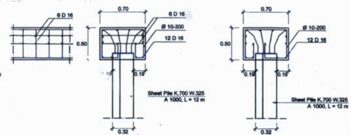
POT. B-B SKALA 1:20
