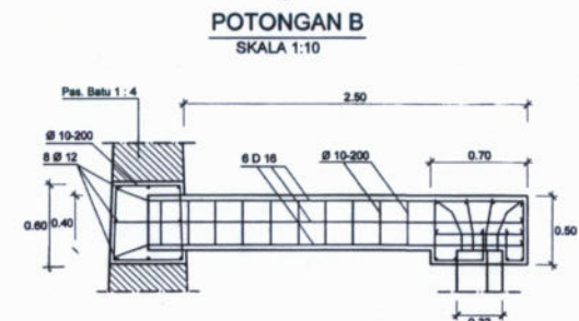
DETAIL PENULANGAN ANGKUR SKALA 1:20
